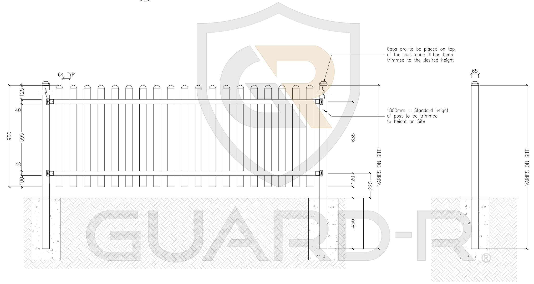
IA PLAN VIEW A-1.0 SCALE: 1:16
